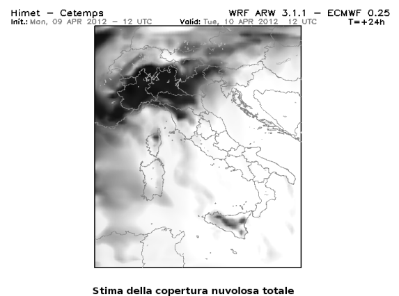
Copertura nuvolosa
