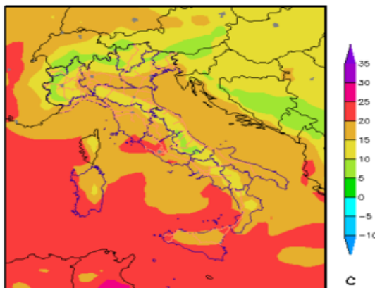
Temperatura a 2m dal suolo
