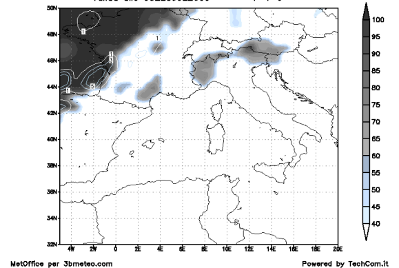
Copertura nuvolosa
