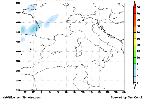
Precipitazione cumulata
