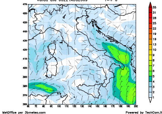
Intensità del vento a 10m dal suolo
