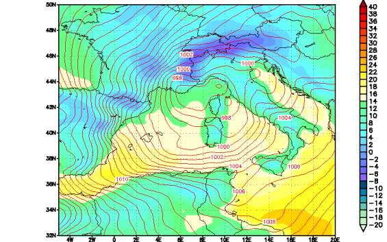
Modello UKMO - Pressione slm (hPa) e Temperatura a 1.5m (C) Run del 00Z09NOV2009 Valida alle 00Z09NOV2009 T=+ 0
