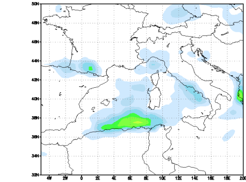
Modello UKMO - Precipitazione cumulata in 6h (mm) Run del 00Z09NOV2009 Valida alle 00Z09NOV2009 T=+ 0
