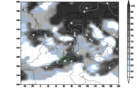
Modello UKMO - Copertura Nuvolosa Totale (%) e Precipitazione 6h (mm) Run del 00Z09NOV2009 Valida alle 00Z09NOV2009 T=+ 0
