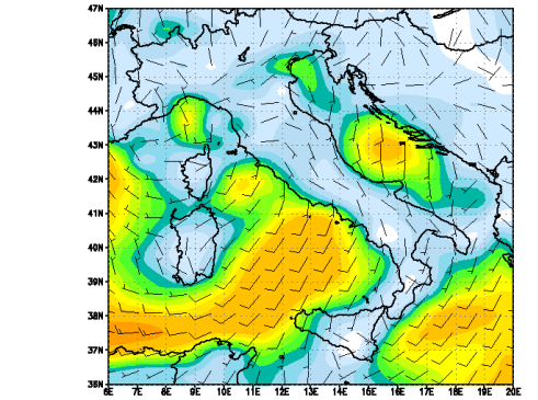
Modello UKMO - Vento a 10 metri (m/s) Run del 00Z09NOV2009 Valida alle 00Z09NOV2009 T=+ 0
