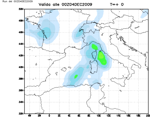
Modello UKMO - Precipitazione cumulata in 6h (mm)
