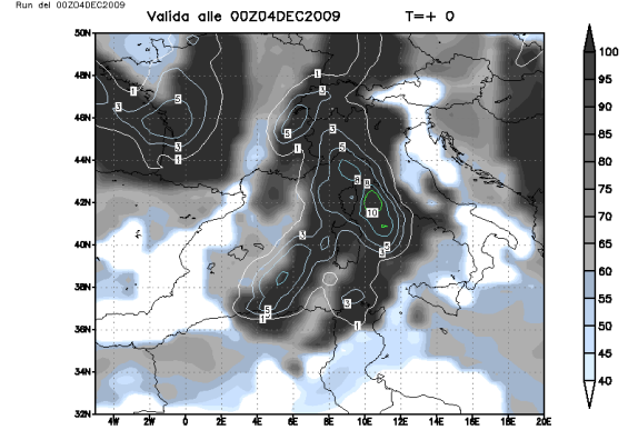
Modello UKMO - Copertura Nuvolosa Totale (%) e Precipitazione 6h (mm)
