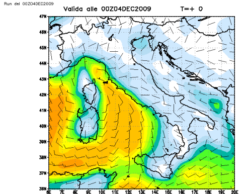
Modello UKMO - Vento a 10 metri (m/s)
