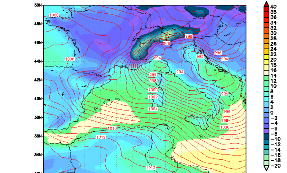
Modello UKMO — Pressione slm (hPa) e Temperatura a 1.5m (C) Run del 00Z31JAN2010
