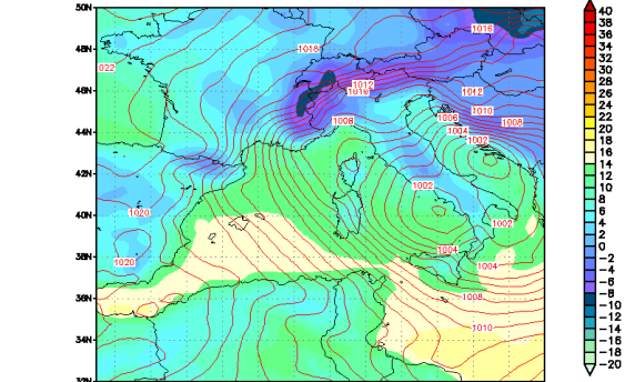
Modello UKMO - Pressione slm (hPa) e Temperatura a 1.5m (C) Run del 00Z07FEB2010 Valida alle 00Z07FEB2010 T=+ 0
