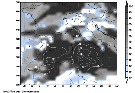
Copertura nuvolosa
