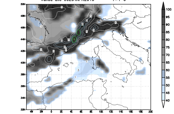
Copertura nuvolosa
