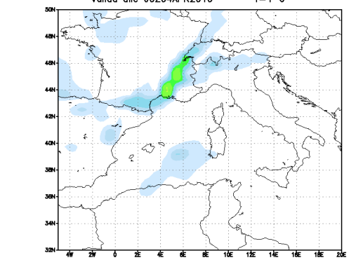
Precipitazione cumulata
