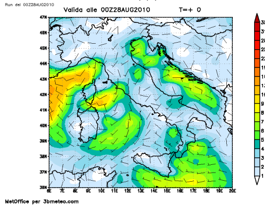
Intensita del vento a 10m dal suolo
