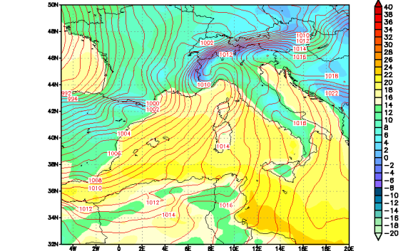
Modello UKMO — Pressione slm (hPa) e Temperatura a 1.5m (C) Run del 00Z31OCT2010
