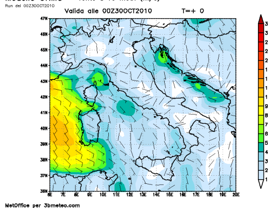
Intensita del vento a 10m dal suolo
