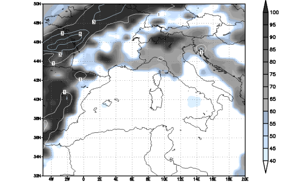
Modello UKMO — Copertura Nuvolosa Totale (%) e Precipitazione 6h (mm) Run del 00Z09JAN2011
