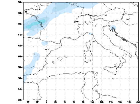
Modello UKMO — Precipitazione cumulata in 6h (mm) Run del 00Z09JAN2011
