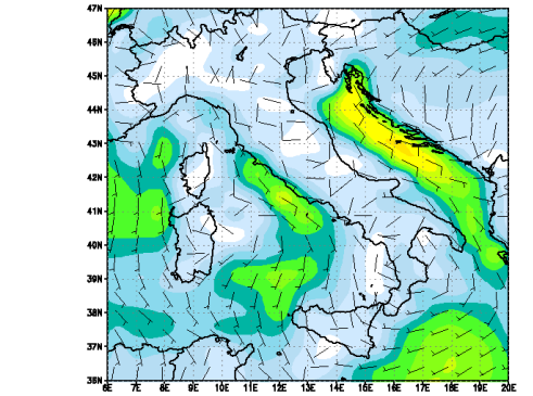
Modello UKMO — Vento a 10 metri (m/s) Run del 00Z09JAN2011
