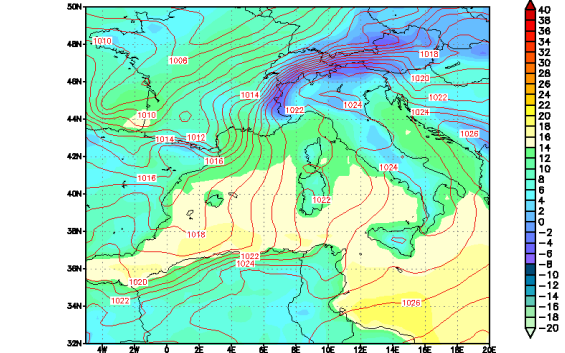
Modello UKMO — Pressione slm (hPa) e Temperatura a 1.5m (C) Run del 00Z09JAN2011
