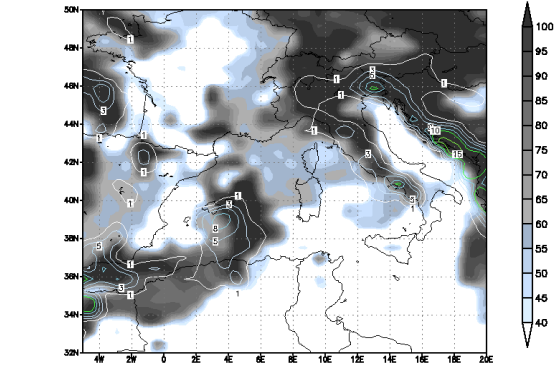
Modello UKMO — Copertura Nuvolosa Totale (%) e Precipitazione 6h (mm) Run del 00Z17FEB2011
