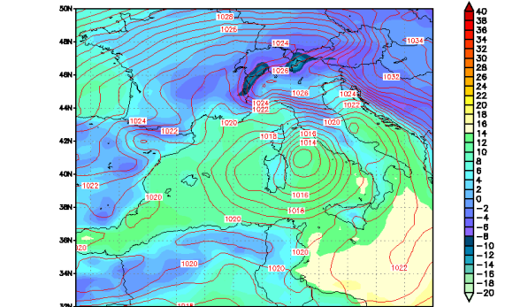
Modello UKMO - Pressione slm (hPa) e Temperatura a 1.5m (C) Run del 00Z03MAR2011 Valida alle 00Z03MAR2011 T=+ 0
