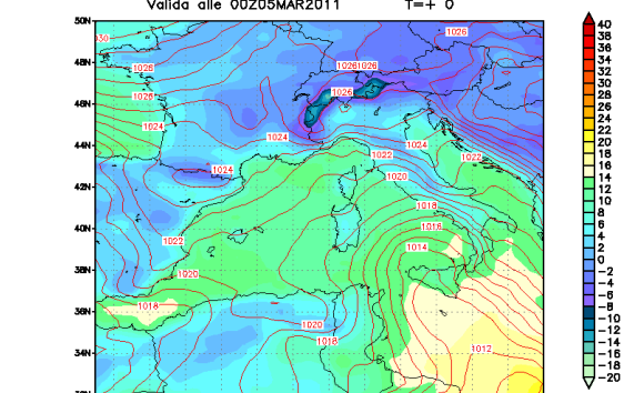
Modello UKMO - Pressione slm (hPa) e Temperatura a 1.5m (C)
