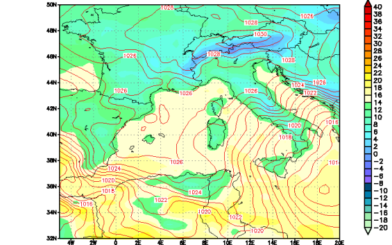
Modello UKMO — Pressione slm (hPa) e Temperatura a 1.5m (C) Run del 00Z06APR2011
