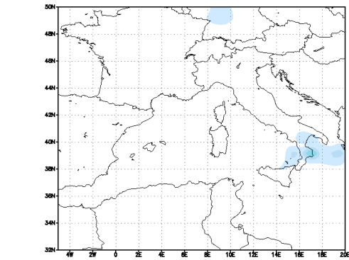
Modello UKMO — Precipitazione cumulata in 6h (mm) Run del 00Z06APR2011
