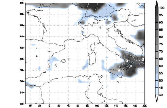
Modello UKMO — Copertura Nuvolosa Totale (%) e Precipitazione 6h (mm) Run del 00Z06APR2011
