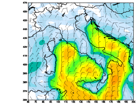
Modello UKMO — Vento a 10 metri (m/s) Run del 00Z06APR2011
