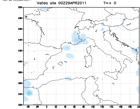
Modello UKMO — Precipitazione cumulata in 6h (mm) Run del 00Z29APR2011
