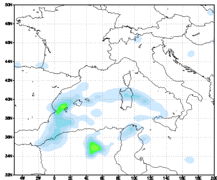
Modello UKMO — Precipitazione cumulata in 6h (mm) Run del 00Z25APR2011 Valida alle 00Z25APR2011 T=+ 0
