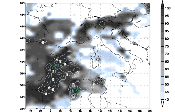
Modello UKMO — Copertura Nuvolosa Totale (%) e Precipitazione 6h (mm) Run del 00Z25APR2011 Valida alle 00Z25APR2011 T=+ 0
