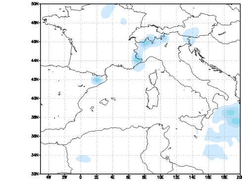
Modello UKMO — Precipitazione cumulata in 6h (mm) Run del 00Z28APR2011
