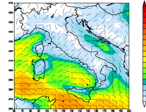
Modello UKMO — Vento a 10 metri (m/s) Run del 00Z25APR2011 Valida alle 00Z25APR2011 T=+ 0
