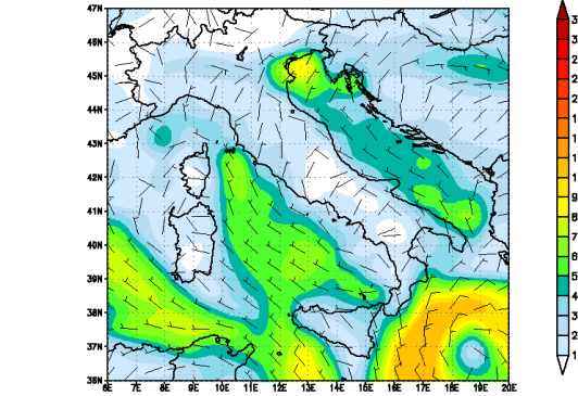
Modello UKMO — Vento a 10 metri (m/s) Run del 00Z28APR2011
