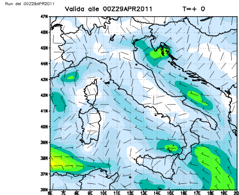
Modello UKMO — Vento a 10 metri (m/s) Run del 00Z29APR2011
