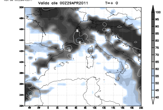
Modello UKMO — Copertura Nuvolosa Totale (%) e Precipitazione 6h (mm) Run del 00Z29APR2011
