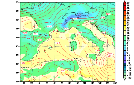
Modello UKMO — Pressione slm (hPa) e Temperatura a 1.5m (C) Run del 00Z28APR2011
