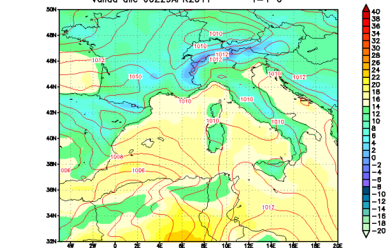
Modello UKMO — Pressione slm (hPa) e Temperatura a 1.5m (C) Run del 00Z29APR2011
