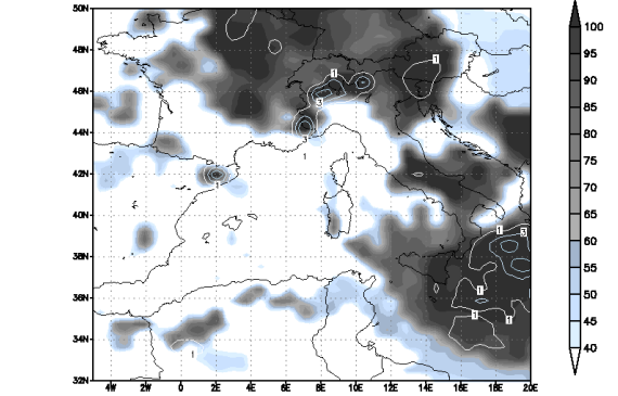
Modello UKMO — Copertura Nuvolosa Totale (%) e Precipitazione 6h (mm) Run del 00Z28APR2011
