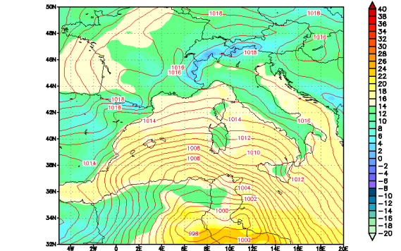
Modello UKMO — Pressione slm (hPa) e Temperatura a 1.5m (C) Run del 00Z25APR2011 Valida alle 00Z25APR2011 T=+ 0
