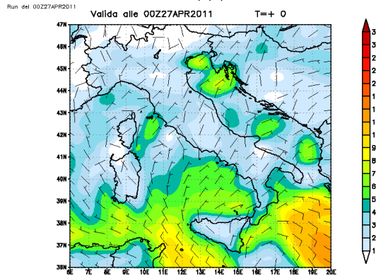
Modello UKMO — Vento a 10 metri (m/s)
