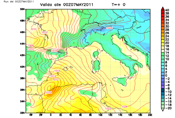
Valida alle 00Z07MAY2011 T=+ 0 MetOffice per 3bmeteo.com Pressione e temperatura al suolo
