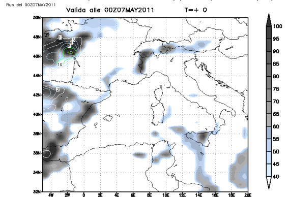
Valida alle 00Z07MAY2011 T=+ 0 MetOffice per 3bmeteo.com Copertura nuvolosa
