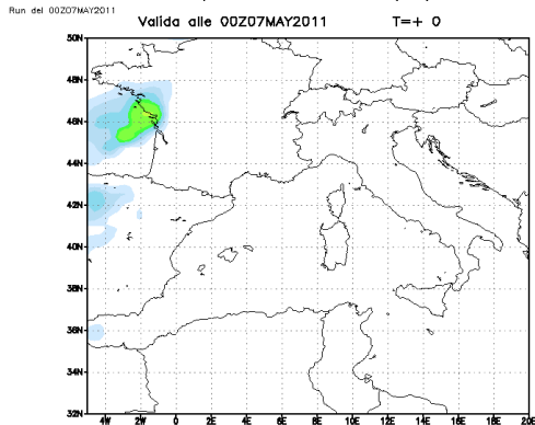
Valida alle 00Z07MAY2011 T=+ 0 MetOffice per 3bmeteo.com Precipitazione cumulata
