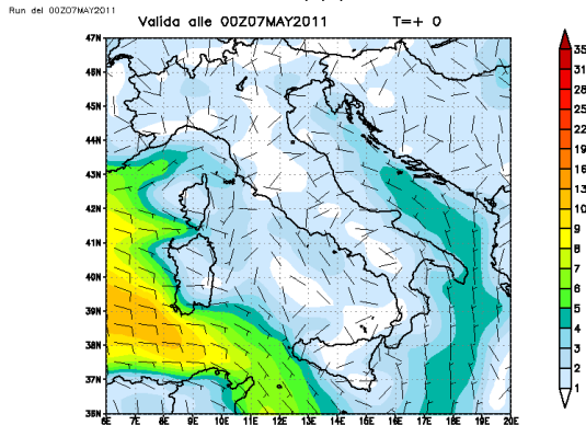
Valida alle 00Z07MAY2011 T=+ 0 MetOffice per 3bmeteo.com Intensita del vento a 10m dal suolo
