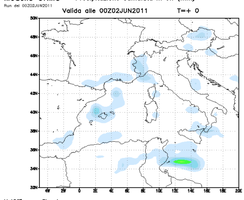
Precipitazione cumulata
