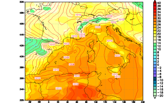
Modello UKMO — Pressione slm (hPa) e Temperatura a 1.5m (C) Run del 00Z13JUL2011
