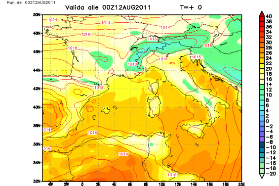
Modello UKMO - Pressione sim (hPa) e Temperatura a 1.5m (C)
