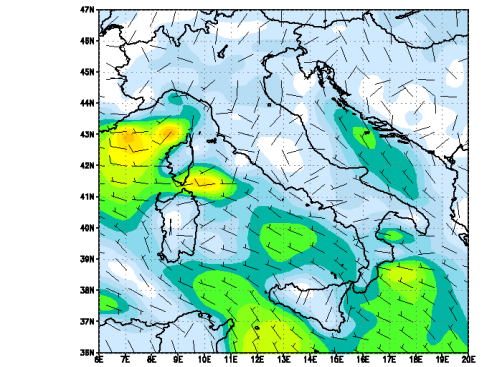
Intensità del vento a 10m dal suolo
