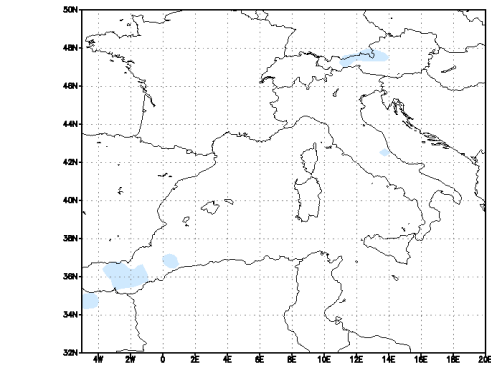
Modello UKMO - Precipitazione cumulata in 6h (mm) Run del 00Z30AUG2011 Valida alle 00Z30AUG2011 T=+ 0
