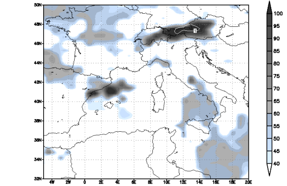
Modello UKMO - Copertura Nuvolosa Totale (%) e Precipitazione 6h (mm) Run del 00Z30AUG2011 Valida alle 00Z30AUG2011 T=+ 0
