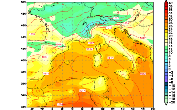
Modello UKMO - Pressione slm (hPa) e Temperatura a 1.5m (C) Run del 00Z30AUG2011 Valida alle 00Z30AUG2011 T=+ 0
