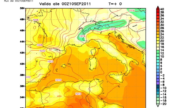
Modello UKMO — Pressione sim (hPa) e Temperatura a 1.5m (C)
