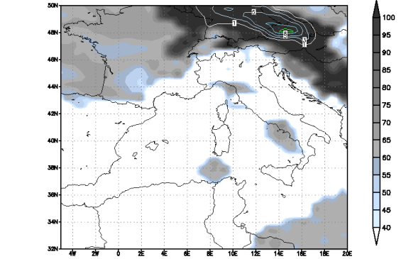
Modello UKMO — Copertura Nuvolosa Totale (%) e Precipitazione 6h (mm) Run del 00Z13OCT2011
