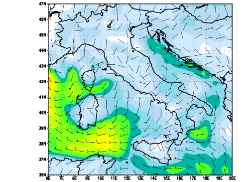
Modello UKMO — Vento a 10 metri (m/s) Run del 00Z13OCT2011
