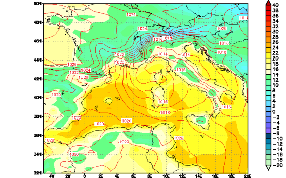
Modello UKMO — Pressione slm (hPa) e Temperatura a 1.5m (C) Run del 00Z13OCT2011
