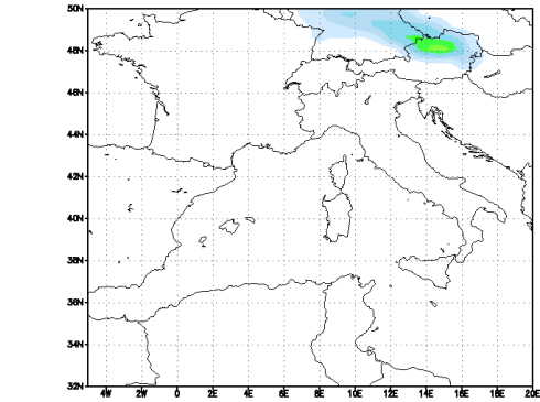
Modello UKMO — Precipitazione cumulata in 6h (mm) Run del 00Z13OCT2011
