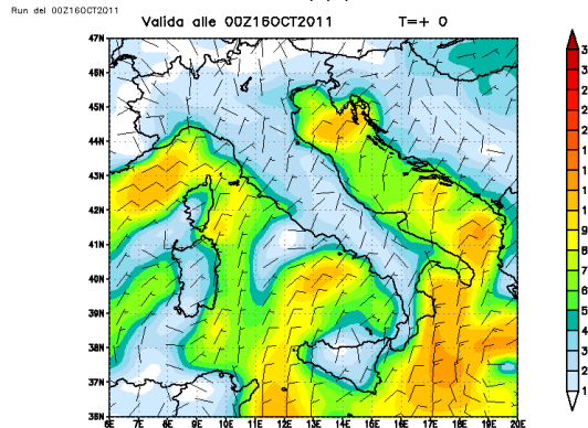
Intensita del vento a 10m dal suolo
