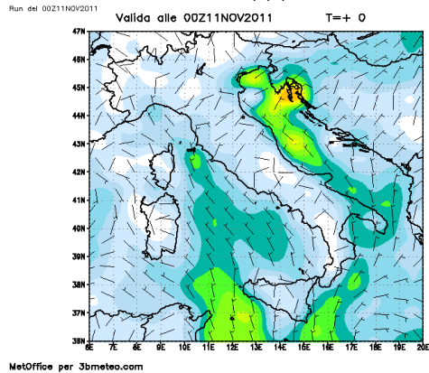
Intensita del vento a 10m dal suolo
