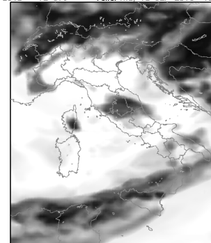
Stima della copertura nuvolosa totale Copertura nuvolosa
