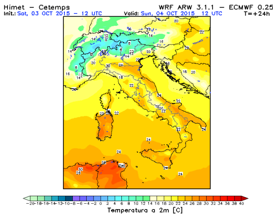
Temperatura a 2m dal suolo
