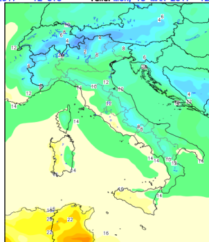
Temperatura a 2m [C]
