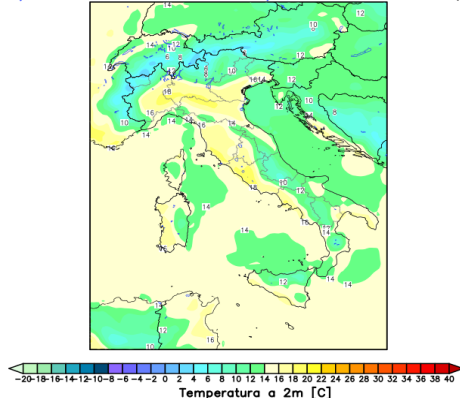
Temperatura a 2m dal suolo
