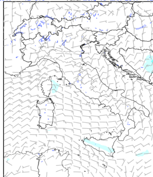
Precipitazione totale [mm/3h] + Vento [nodi]
