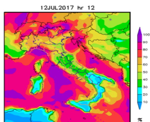
Arpa Lazio - rh - run 20170712 forecast +12h - WRF-ARW 3.5.1 Umidità relativa
