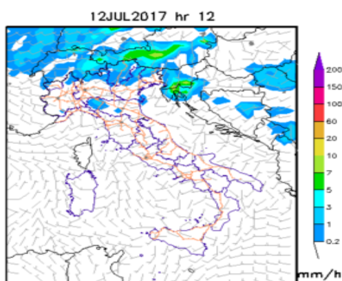
Arpa Lazio - prec - run 20170712 forecast +12h - WRF-ARW 3.5.1 Precipitazione cumulata e vento
