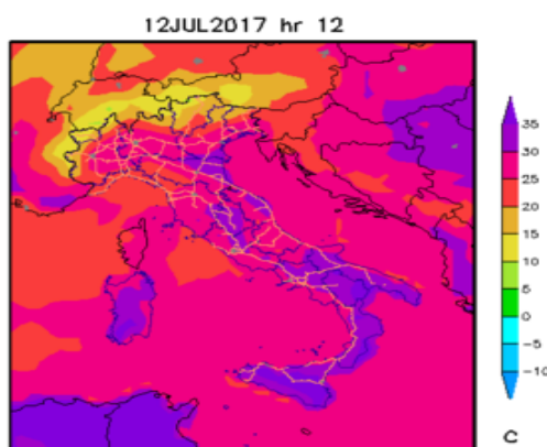
Arpa Lazio - t - run 20170712 forecast +12h - WRF-ARW 3.5.1 Temperatura a 2m dal suolo
