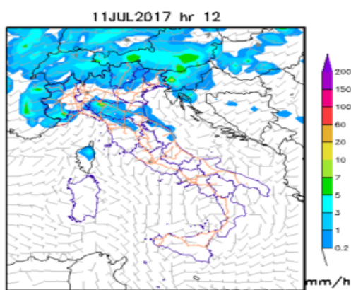
Precipitazione cumulata e vento
