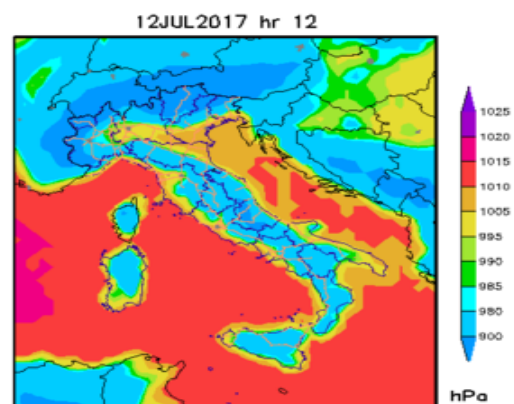
Arpa Lazio - p - run 20170712 forecast +12h - WRF-ARW 3.5.1 Pressione
