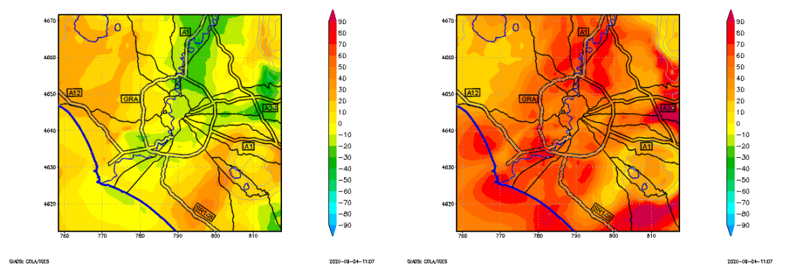
NO_2 - Valore massimo
