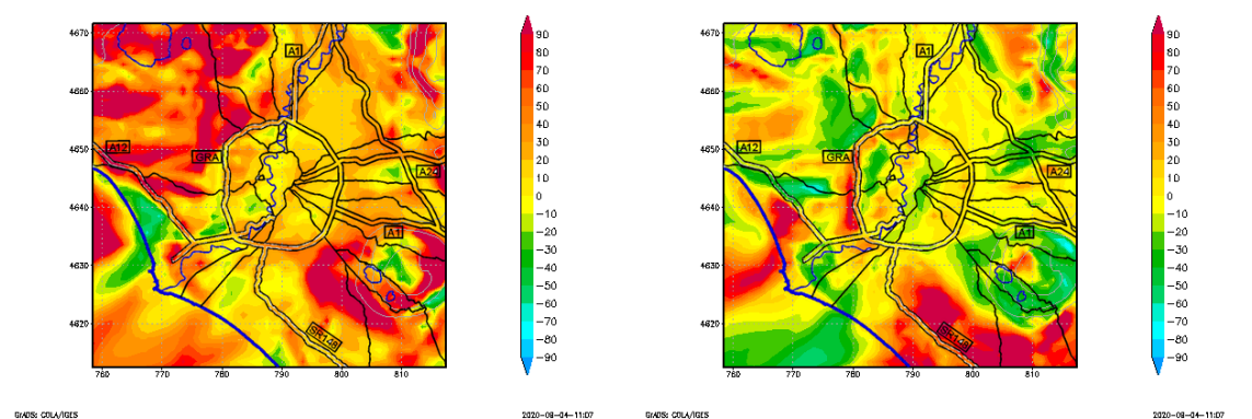
O_3 - Valore massimo
